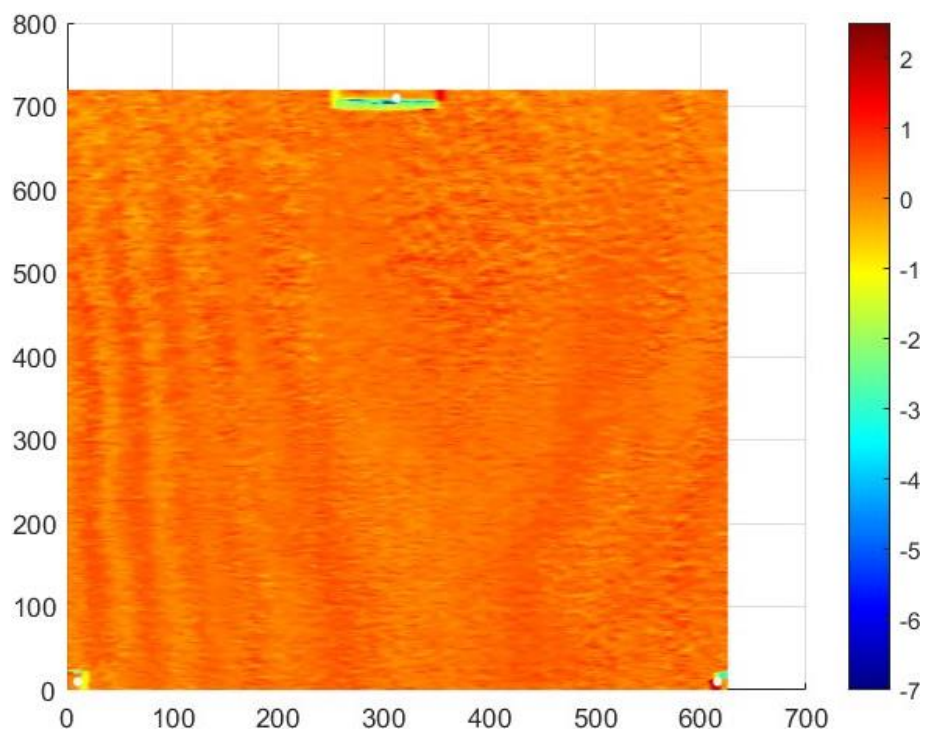
Abbildung 8: Probekörper 1 – Aufsicht, 120.000 Zyklen (Achsenbeschriftungen entsprechen Messpunkten des Lasers, Millimetereinteilung (Höhe auf Probe) an Farbskala)
