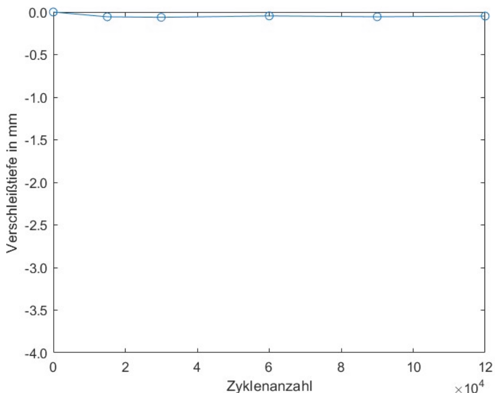
Abbildung 13: Probekörper 3 – Median mittlere Verschleißtiefe V_{m,3} : 0,1 mm (120.000 Zyklen)
