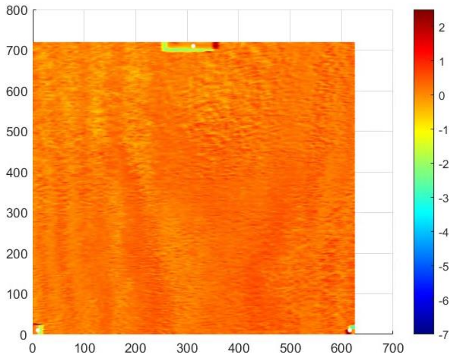
Abbildung 7: Probekörper 1 – Aufsicht, 15.000 Zyklen (Achsenbeschriftungen entsprechen Messpunkten des Lasers, Millimetereinteilung (Höhe auf Probe) an Farbskala)
