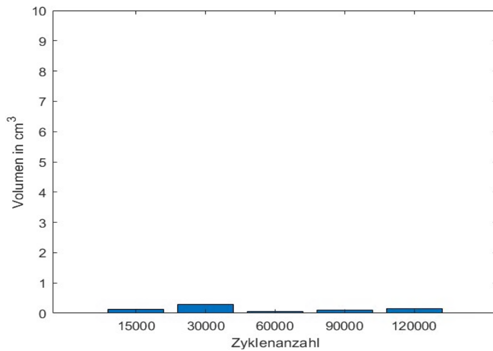
Abbildung 21: Probekörper 3: Verschleißvolumen des gesamten Belastungsbereichs in Abhängigkeit von den Belastungszyklen; V_{\text{Vol},3} : 0,3 cm 3 (120.000 Zyklen)
