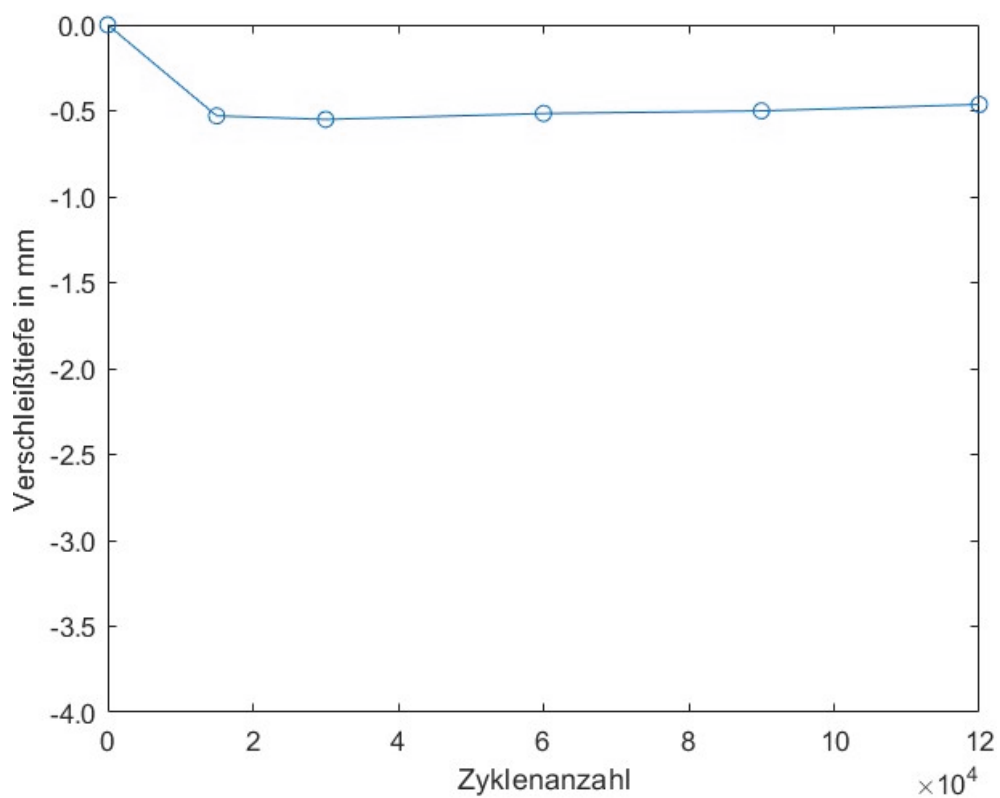
Abbildung 6: Probekörper 1 – Median maximale Verschleißtiefe V_{max,1} : 0,5 mm (120.000 Zyklen)
