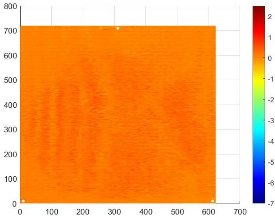
Abbildung 15: Probekörper 3 – Aufsicht, 15.000 Zyklen (Achsenbeschriftungen entsprechen Messpunkten des Lasers, Millimetereinteilung (Höhe auf Probe) an Farbskala)
