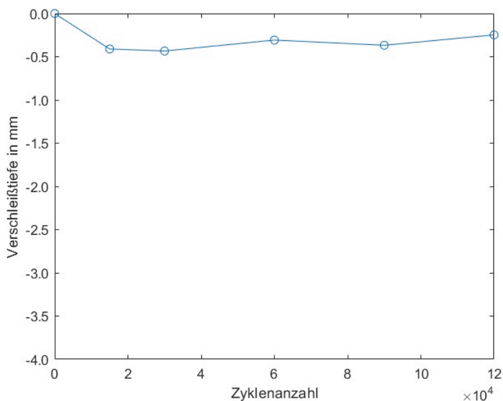
Abbildung 14: Probekörper 3 – Median maximale Verschleißtiefe V_{max,3} : 0,3 mm (120.000 Zyklen)
