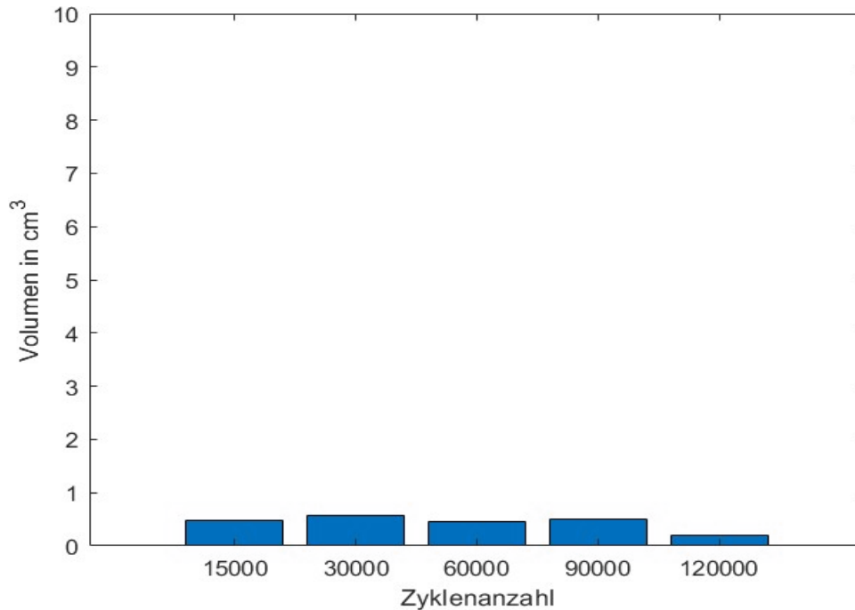
Abbildung 17: Probekörper 1: Verschleißvolumen des gesamten Belastungsbereichs in Abhängigkeit von den Belastungszyklen; V_{\text{Vol},1} : 0,4 \text{ cm}^3 (120.000 Zyklen)
