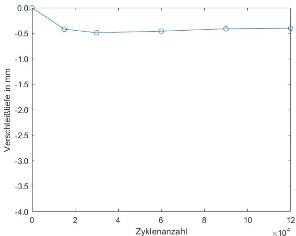
Abbildung 10: Probekörper 2 – Median maximale Verschleißtiefe V_{max,2} : 0,4 mm (120.000 Zyklen)
