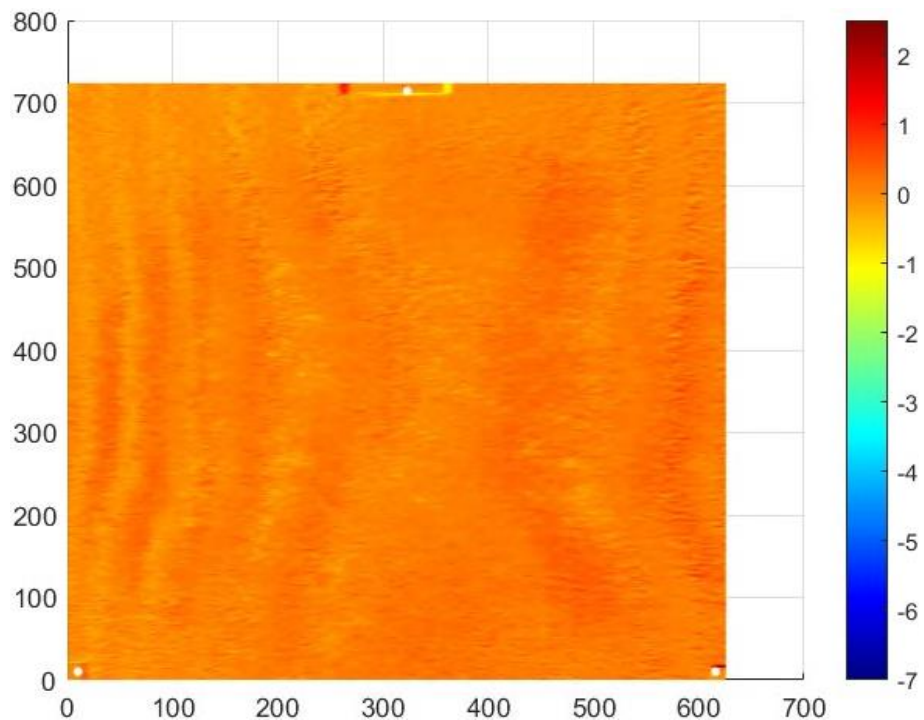
Abbildung 12: Probekörper 2 – Aufsicht, 120.000 Zyklen (Achsenbeschriftungen entsprechen Messpunkten des Lasers, Millimetereinteilung (Höhe auf Probe) an Farbskala)
