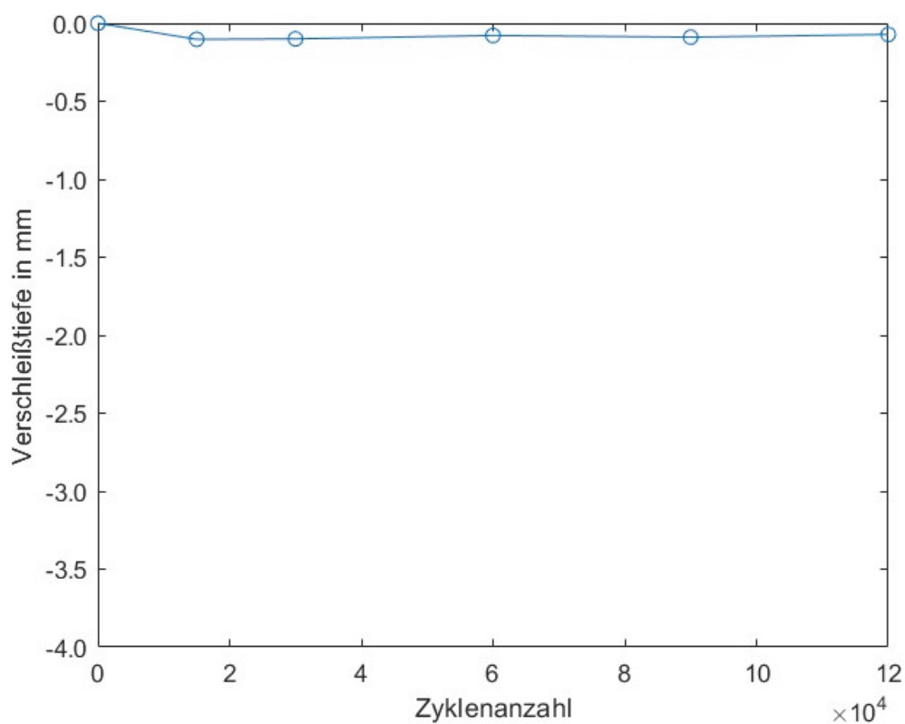
Abbildung 5: Probekörper 1 – Median mittlere Verschleißtiefe V_{m,1} : 0,1 mm (120.000 Zyklen)
