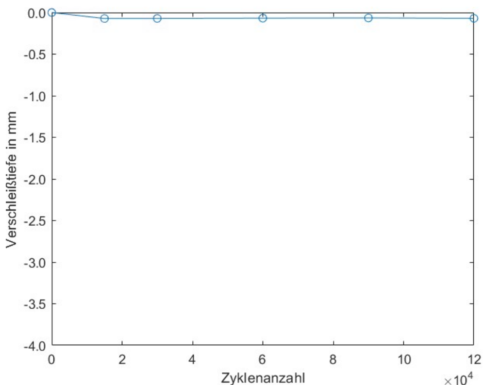
Abbildung 9: Probekörper 2 – Median mittlere Verschleißtiefe V_{m,2} : 0,1 mm (120.000 Zyklen)
