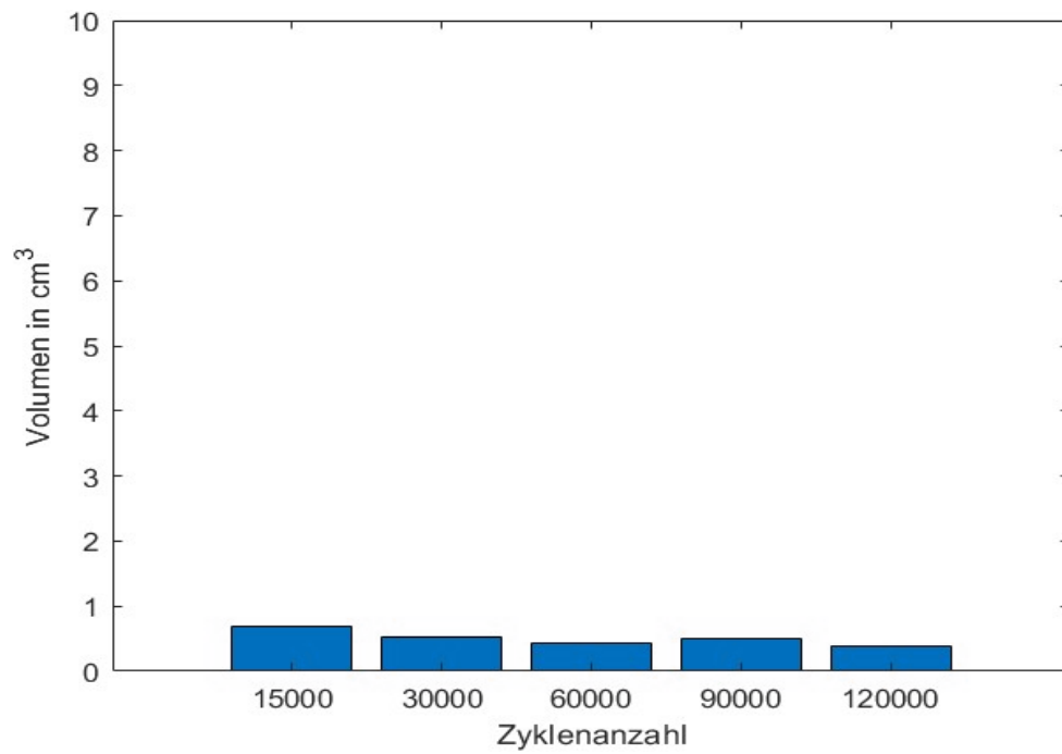
Abbildung 19: Probekörper 2: Verschleißvolumen des gesamten Belastungsbereichs in Abhängigkeit von den Belastungszyklen; V_{\text{Vol},2} : 0,5 cm 3 (120.000 Zyklen)
