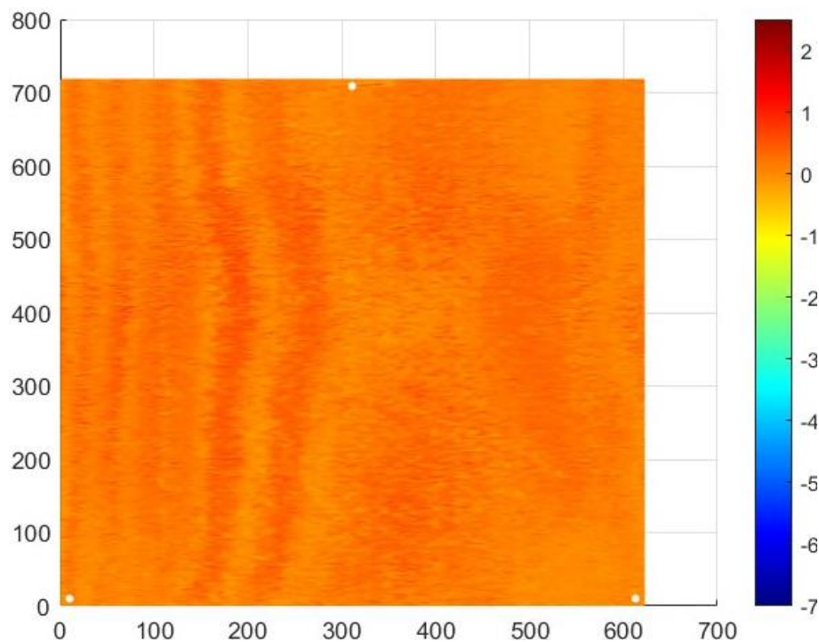
Abbildung 16: Probekörper 3 – Aufsicht, 120.000 Zyklen (Achsenbeschriftungen entsprechen Messpunkten des Lasers, Millimetereinteilung (Höhe auf Probe) an Farbskala)
